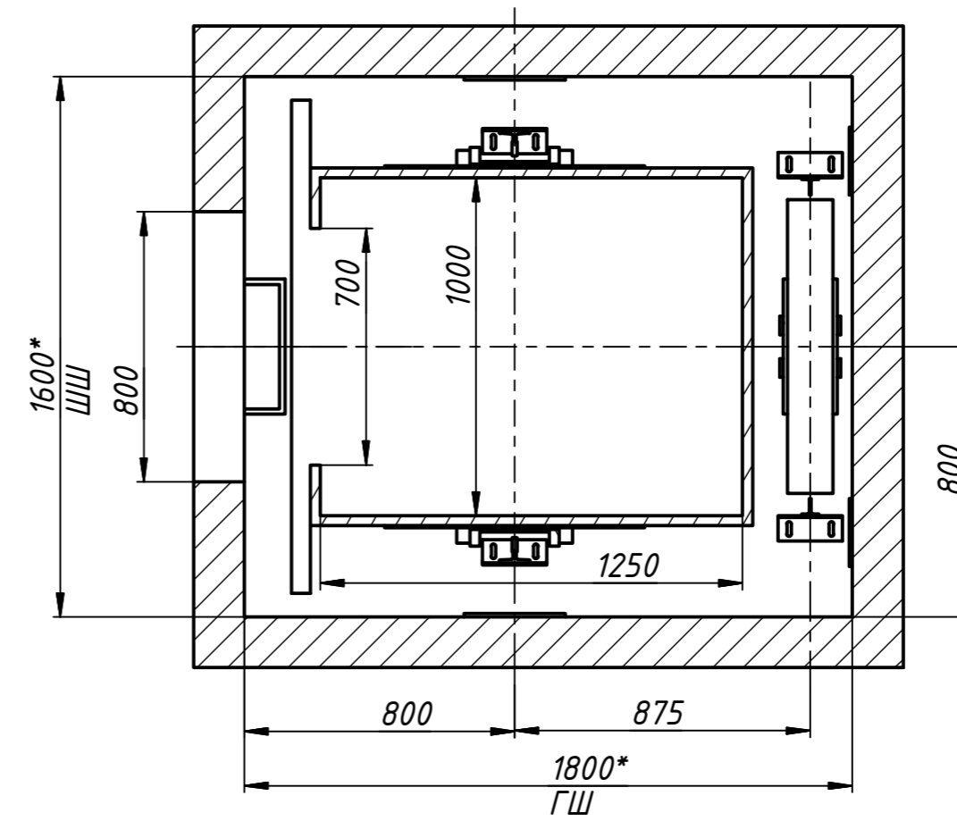
А-А (1:20)
